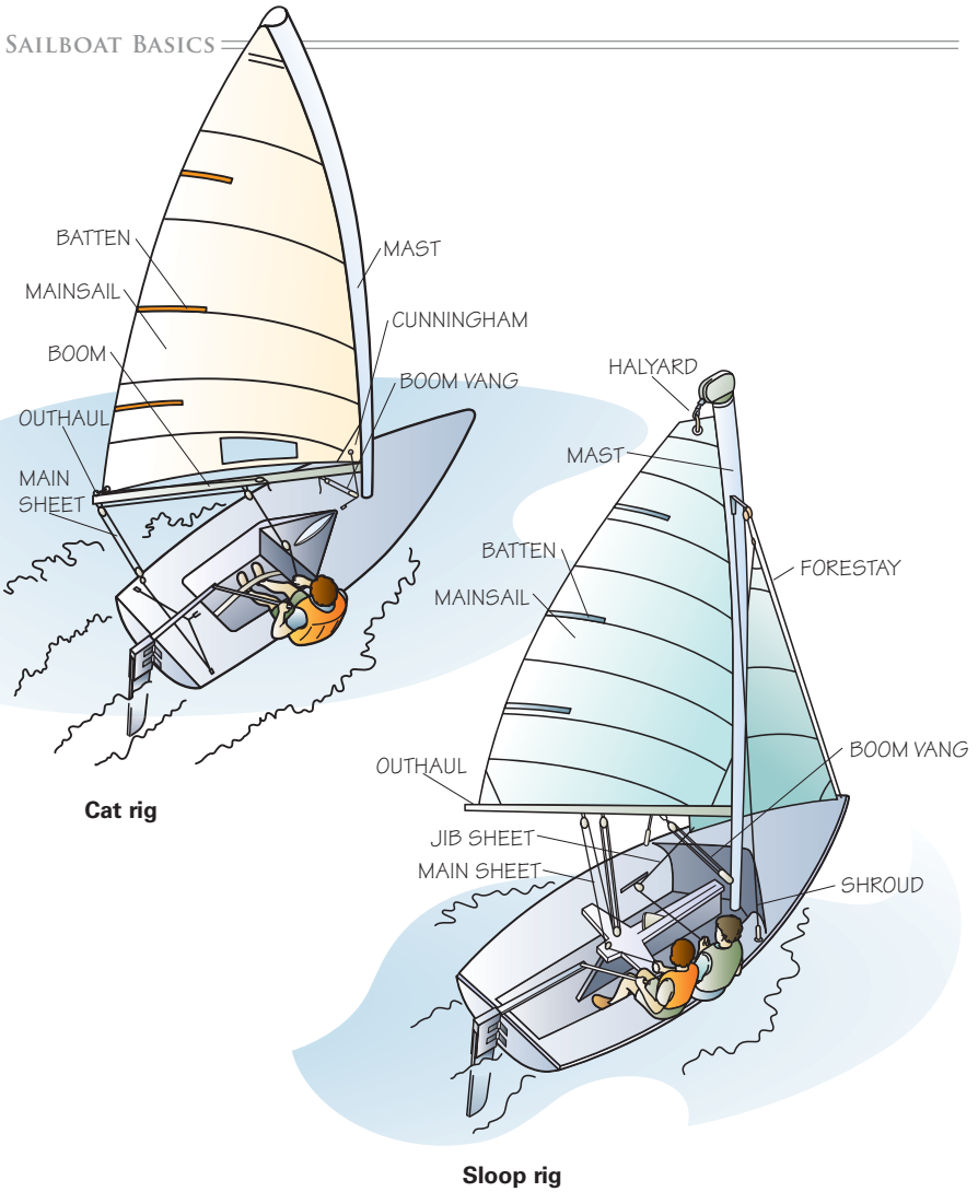
Sloop rig
